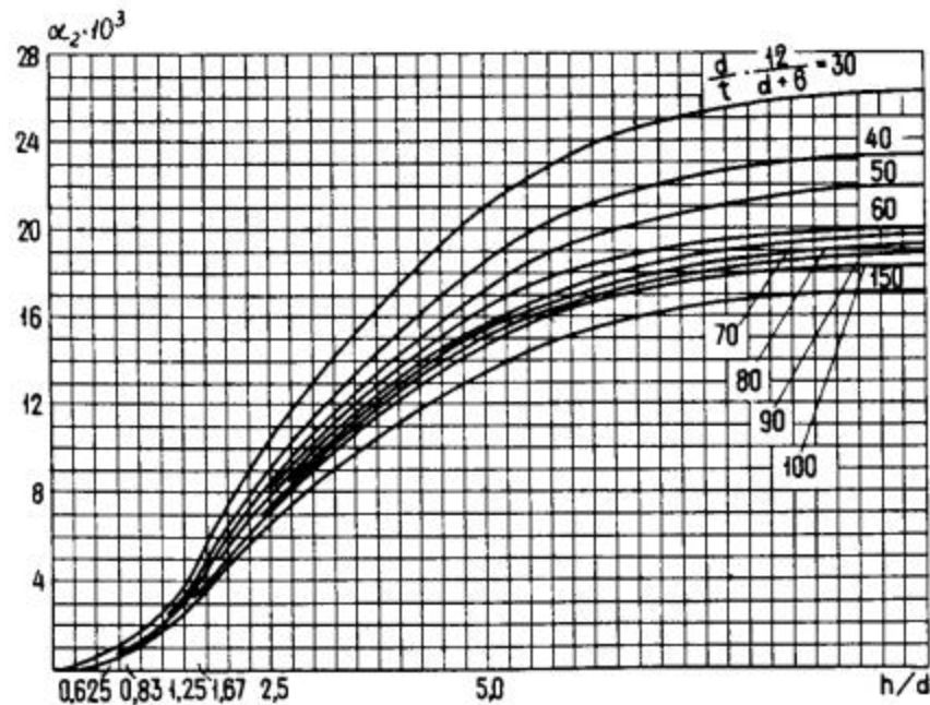
Черт. 5. Значений коэффициента \alpha_2
