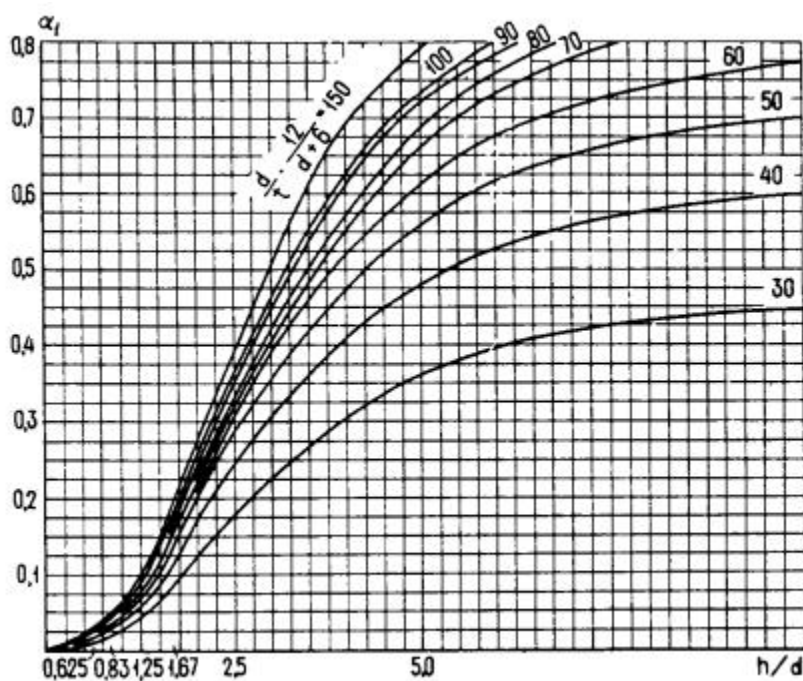
Черт. 4. Значения коэффициента a_1
