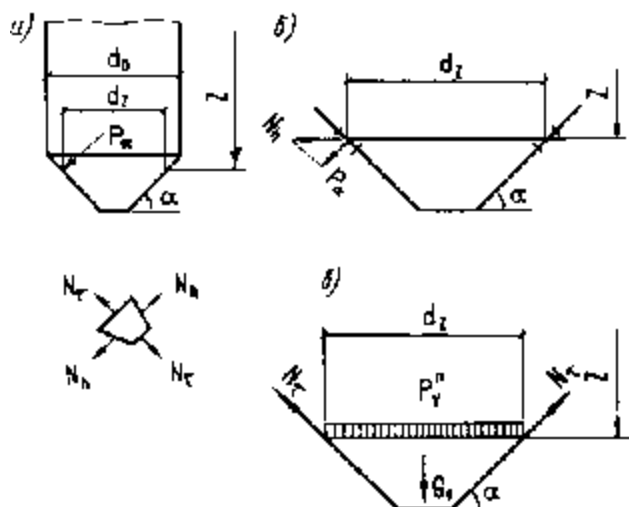
Черт. 7. Расчетные схемы конической воронки
