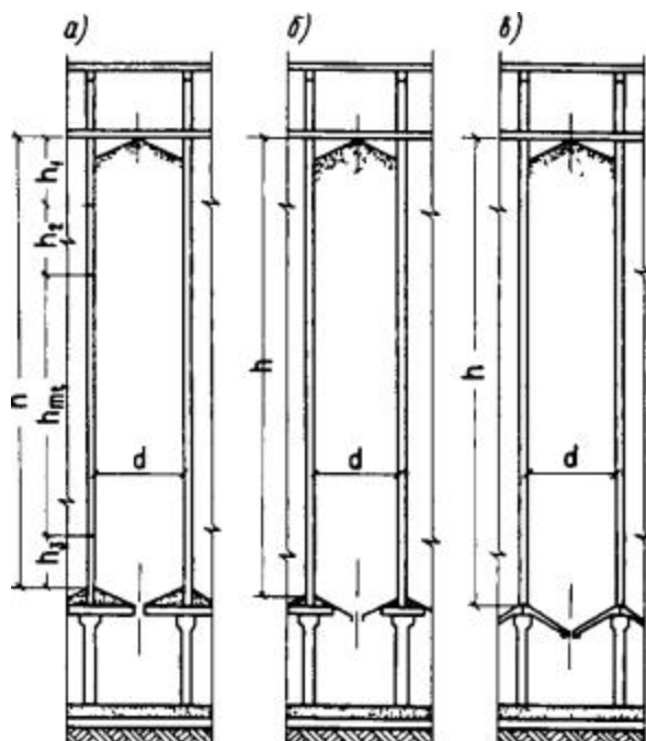
Черт. 1. Разрезы силосов
