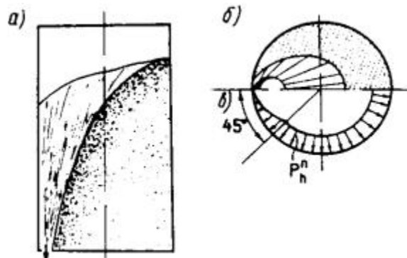
Черт. 3. Пристенный выпуск зерна
