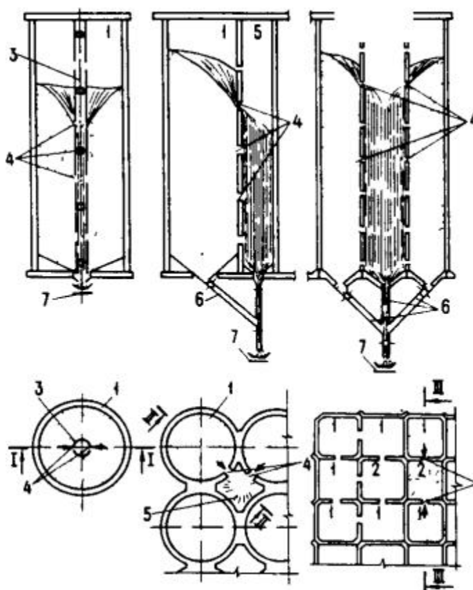
Черт. 2. Выпуск сыпучего материала из силоса
