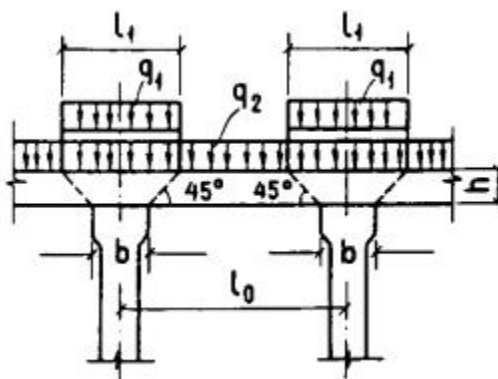
Черт. 8. Передача нагрузки от балки на колонну
